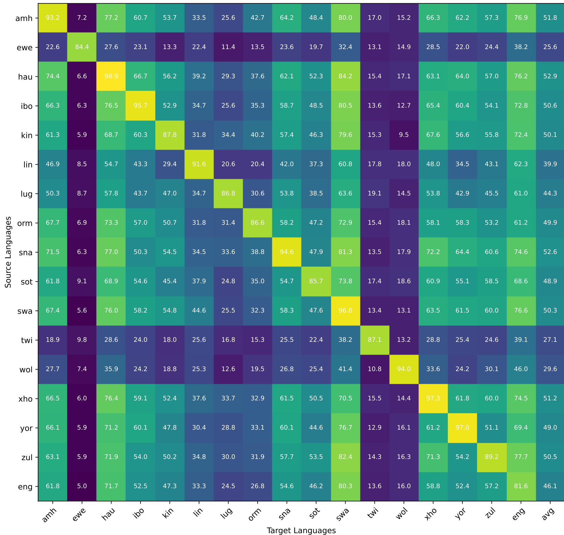
AfriTeVa V2 Intent Detection
